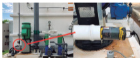
FIGURA 5. Salida al Scrubber (izquierda) y medición de H 2 S con el quipo OdaLog.
